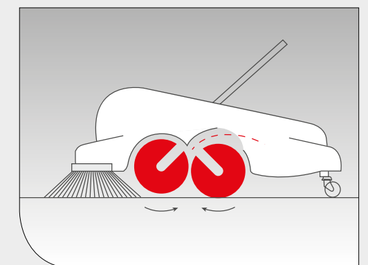
Die gegenläufigen Kehrwalzen des Doppelwalzensystems befördern Kehr gut in den Behälter.
