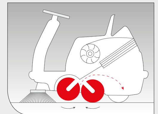
Die gegenläufigen Kehrwalzen des Doppelwalzensystems befördern Kehrut in den Behälter.
