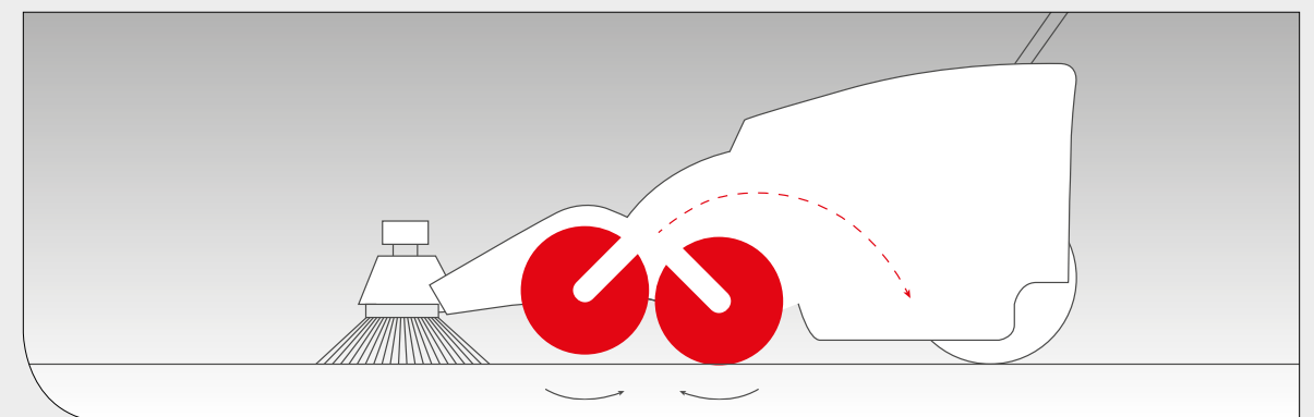
Durch das Doppelwalzensystem wird das Kehrgut mit Hilfe der gegenläufig rotierenden Kehrwalzen aufgenommen und in den Behälter befördert.
