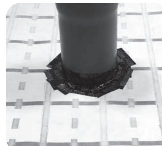
Runde Durchdringung luftdicht verklebt innen
